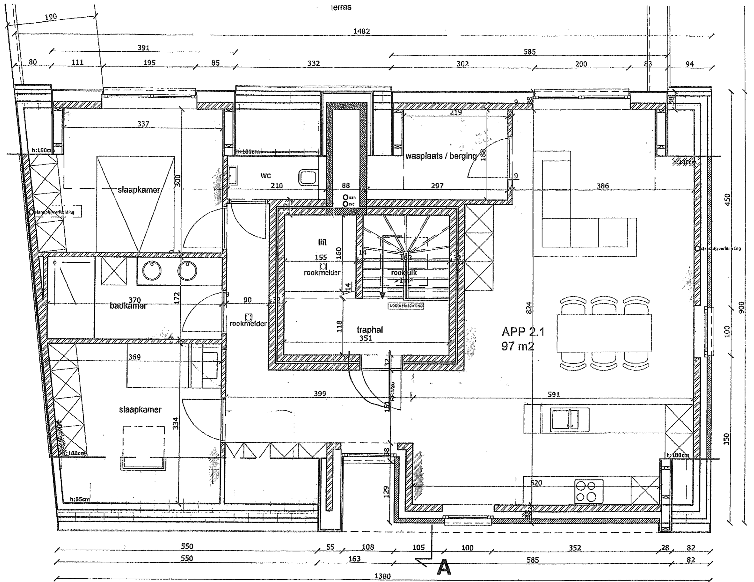
tweede verdieping 1/50
